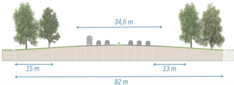
Basis dwarsprofiel verbreding A2 incl. Parkway
